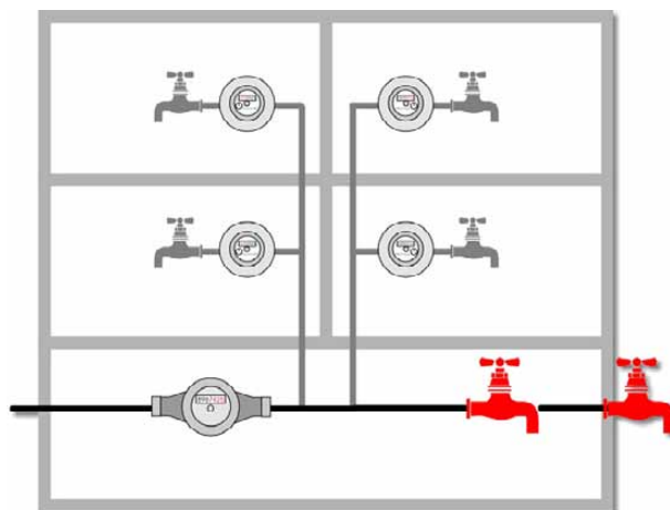
Nicht erfasste Zapfstellen führen zu Differenzen. Typisch dafür sind Garten- und Garagenleitungen. Ist der Verbrauch dieser Zapfstellen gering, darf auf den Einbau von Zählern allerdings verzichtet werden.
