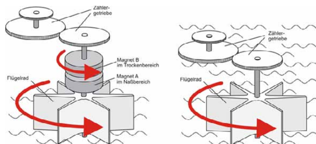
Wohnungswasserzähler sind in der Regel Trockenläufer mit Magnetkupplung (links). Die Hauptzähler der Wasserversorgungsunternehmen sind dagegen Nassläufer (rechts). Nassläufer sind genauer, können aber in Wohnungen nicht eingesetzt werden, weil durch Lichteinfall (Sonne) eine Algenbildung im Schauglas nicht vermeidbar wäre. Diese Lichteinwirkung wird bei Hauswasserzählern durch einen abdunkelnden Schutzdeckel verhindert.
