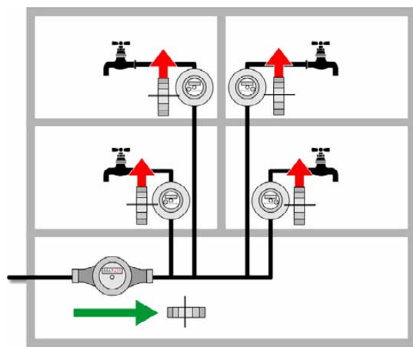
Bei vertikalem Einbau der Wohnungswasserzähler liegt die Flügelradachse horizontal. Dadurch ist die Anlaufempfindlichkeit um ein paar Prozent geringer, als bei dem fast immer horizontal eingebauten Hauptzähler.
